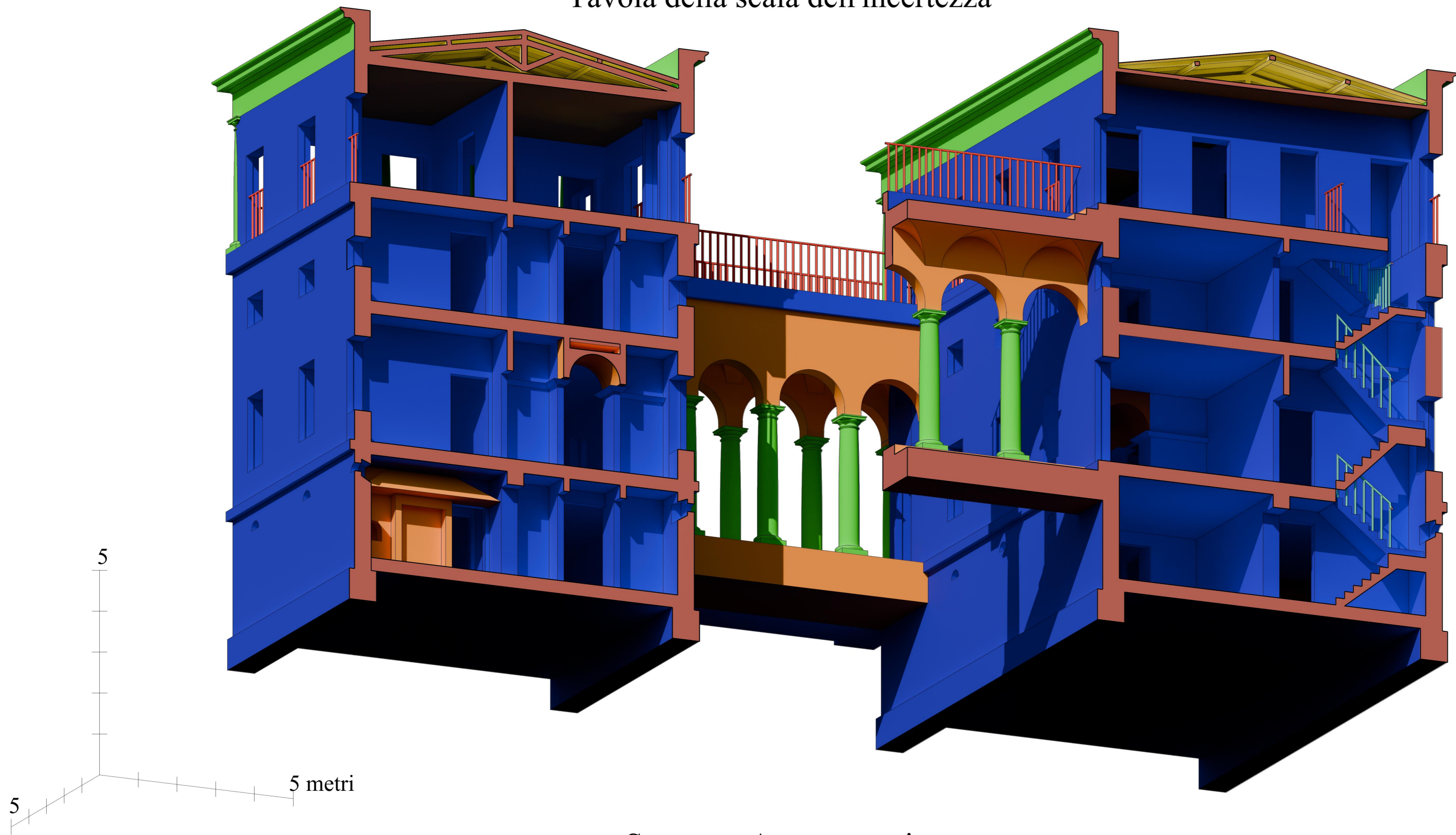
Spaccato Assonometrico
