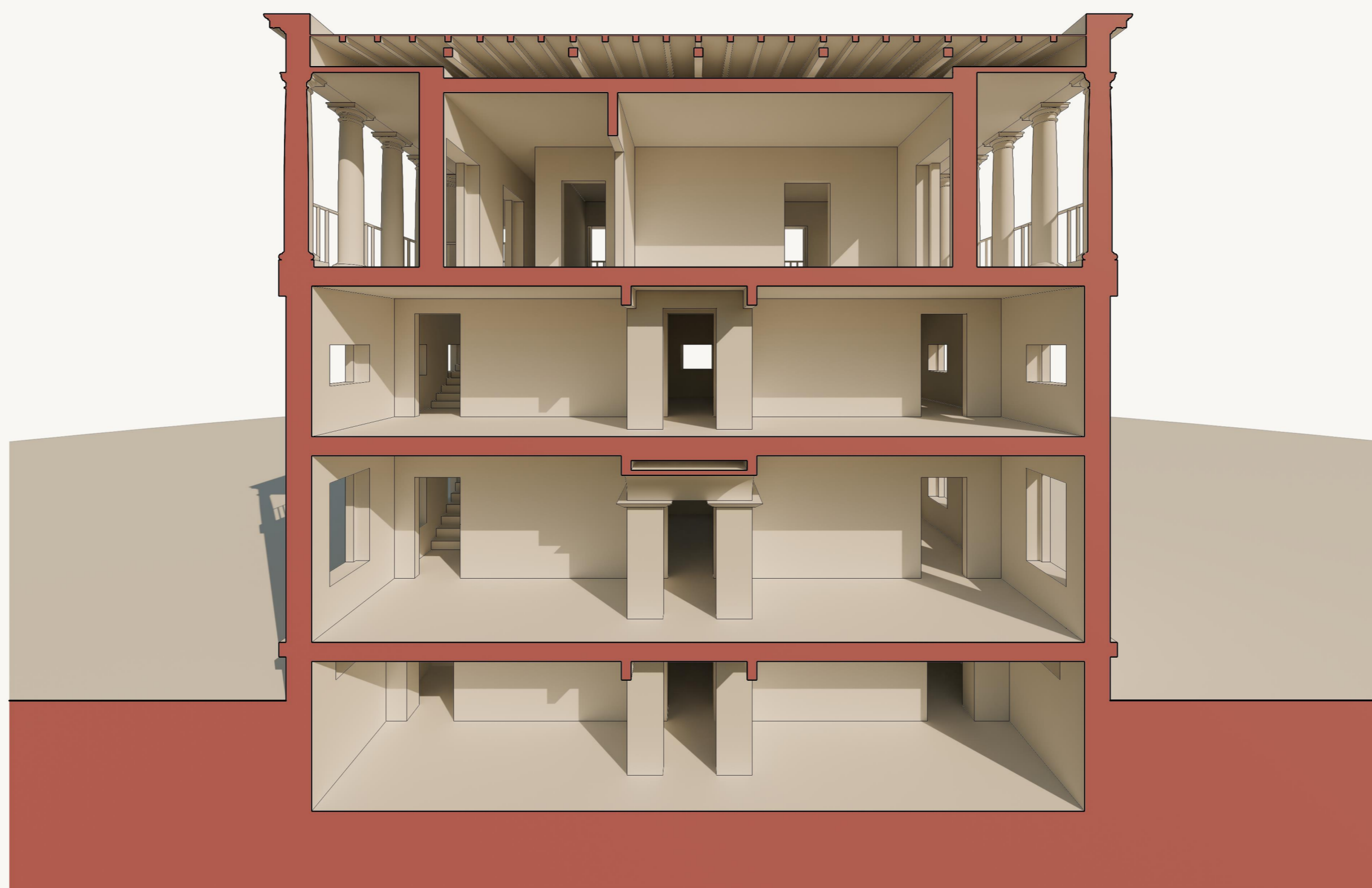
Sezione Trasversale B-B' Prospettica
