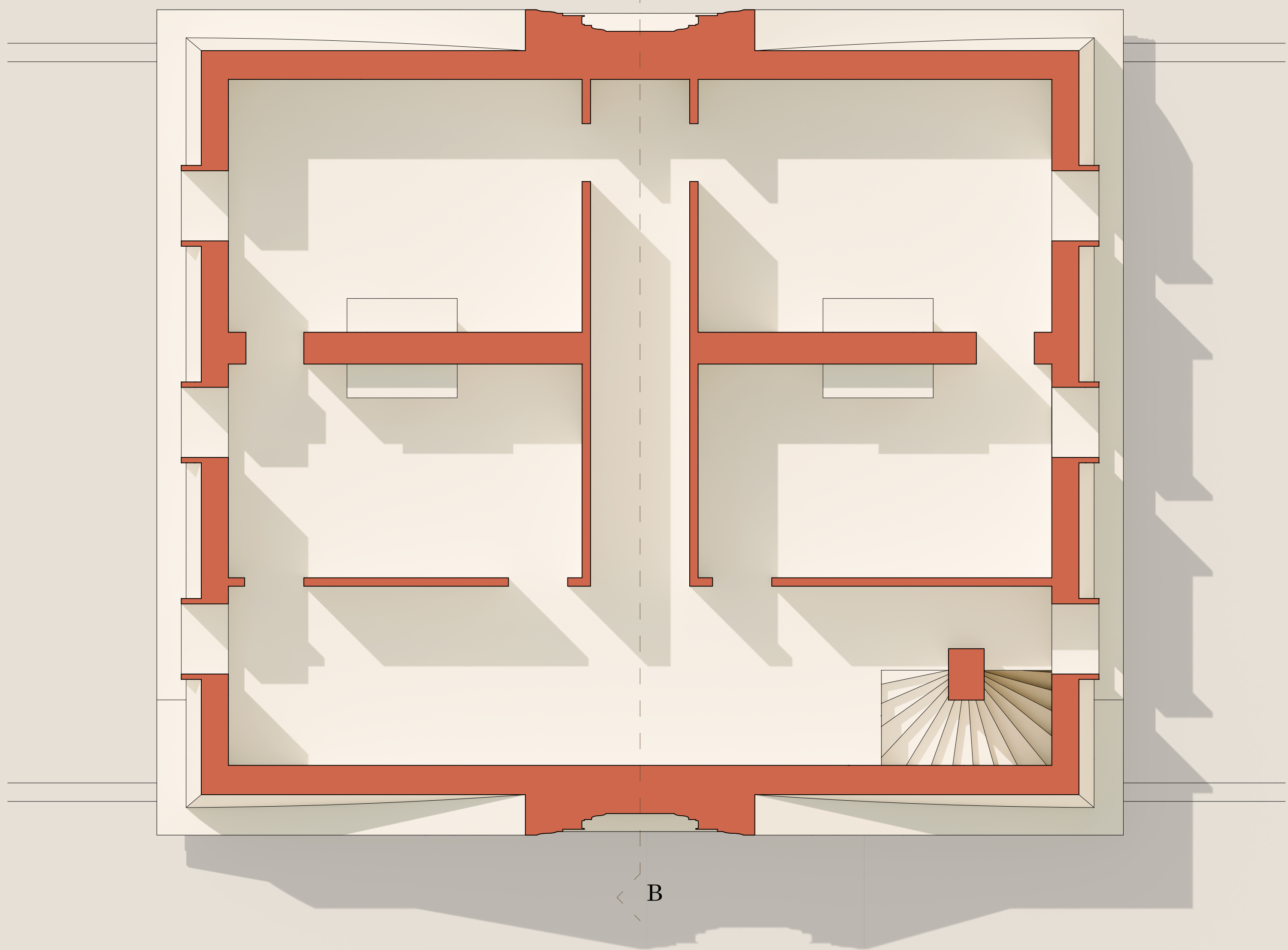
Pianta secondo piano
