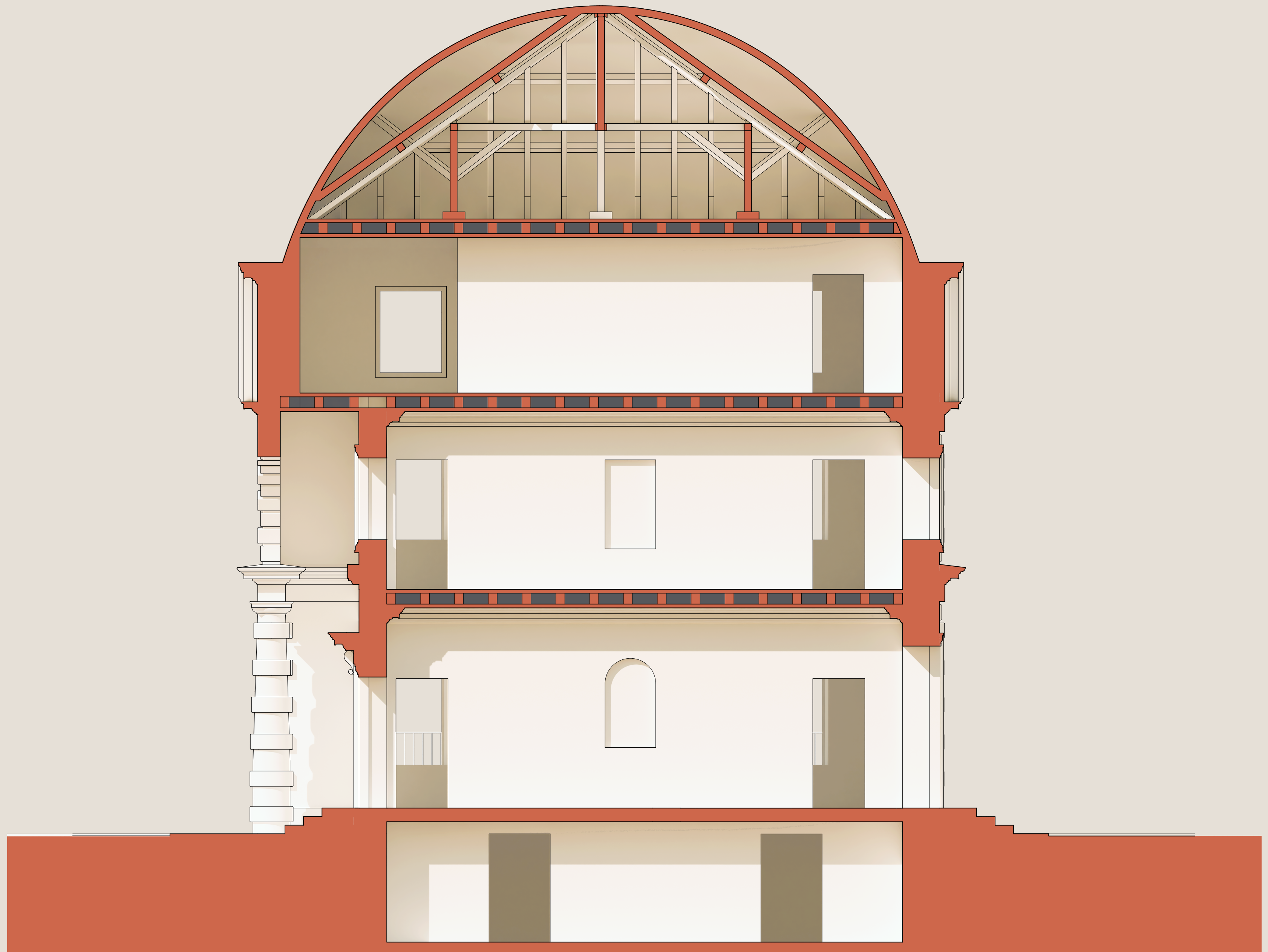
Sezione trasversale B-B'
