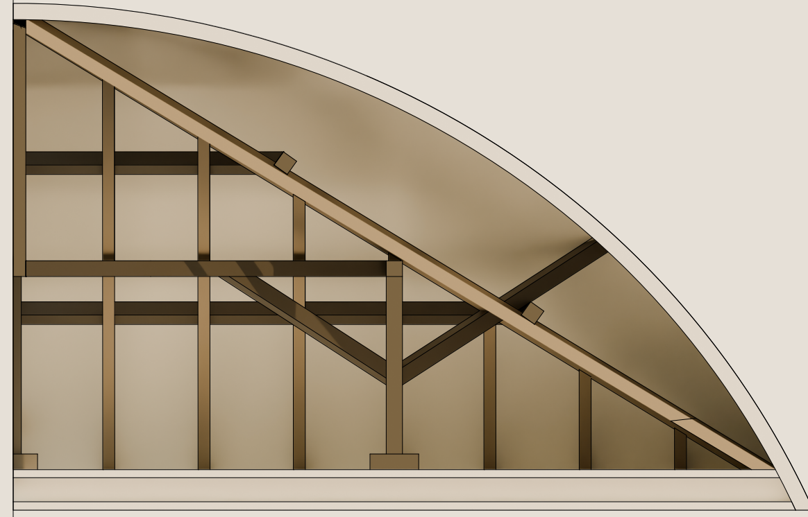
Dettaglio ortogonale della copertura
