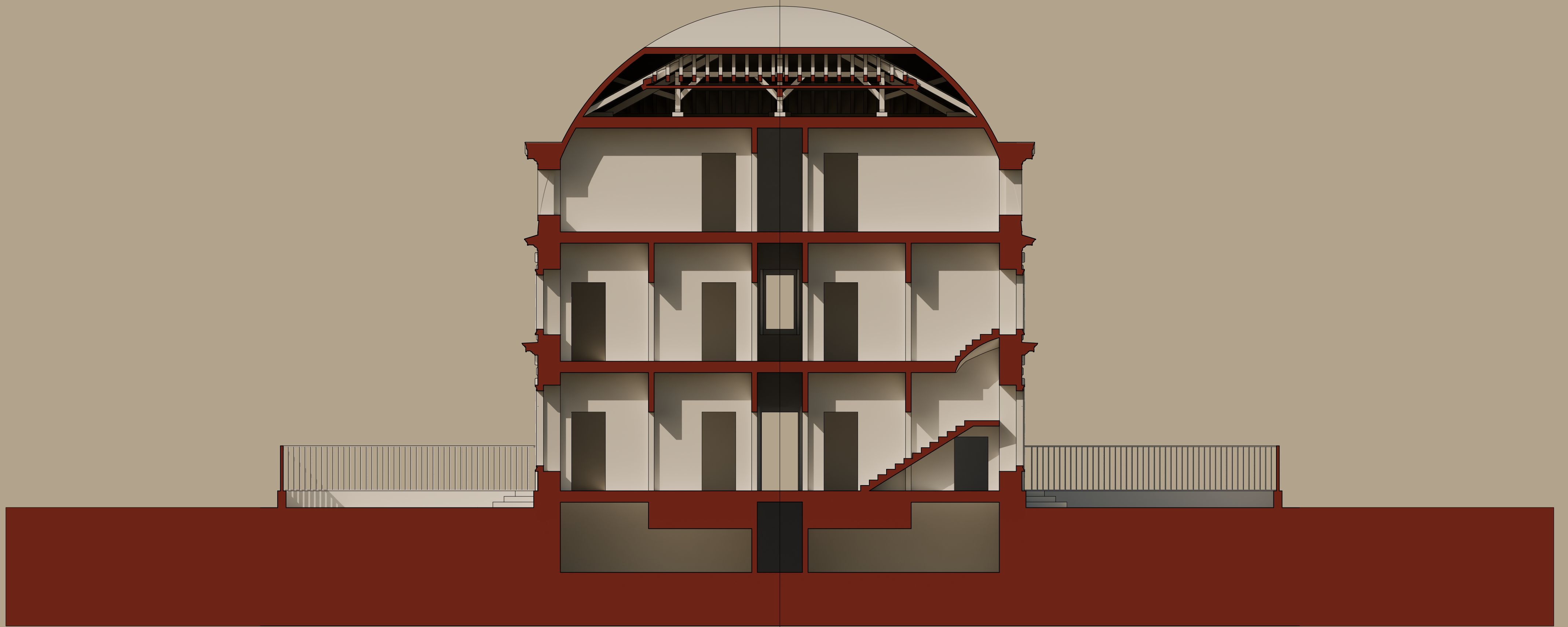
Sezione B-B
