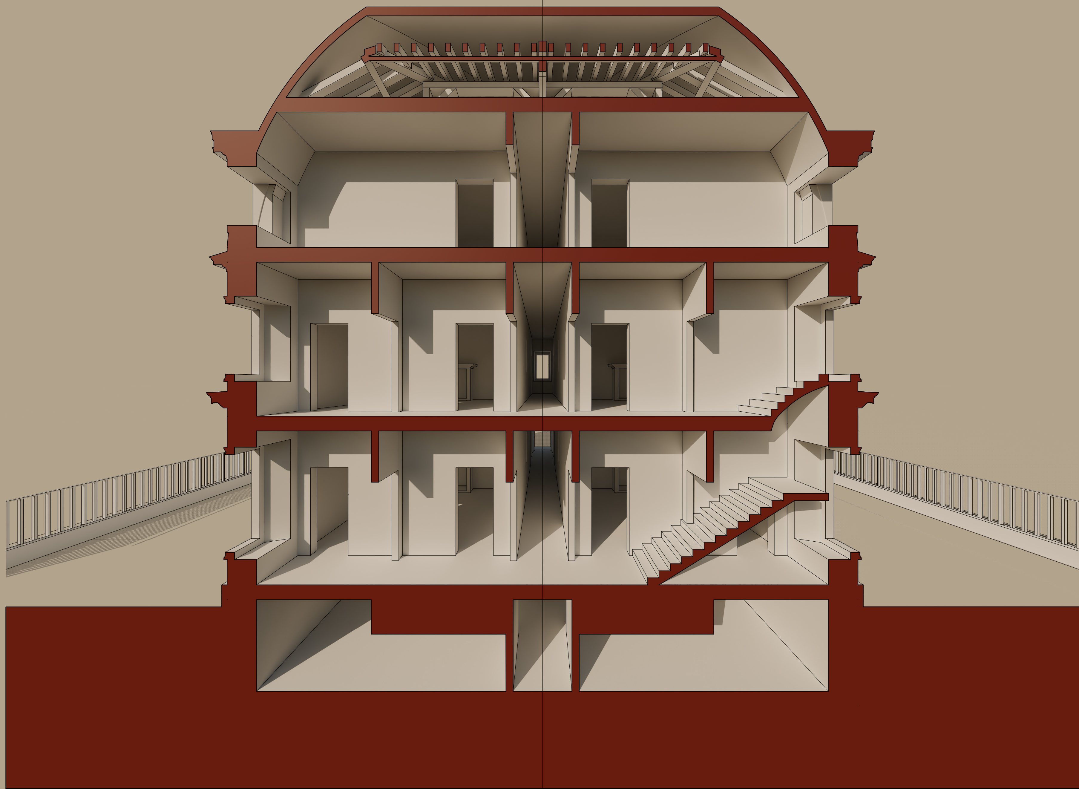
Sezione Prospettica B-B
