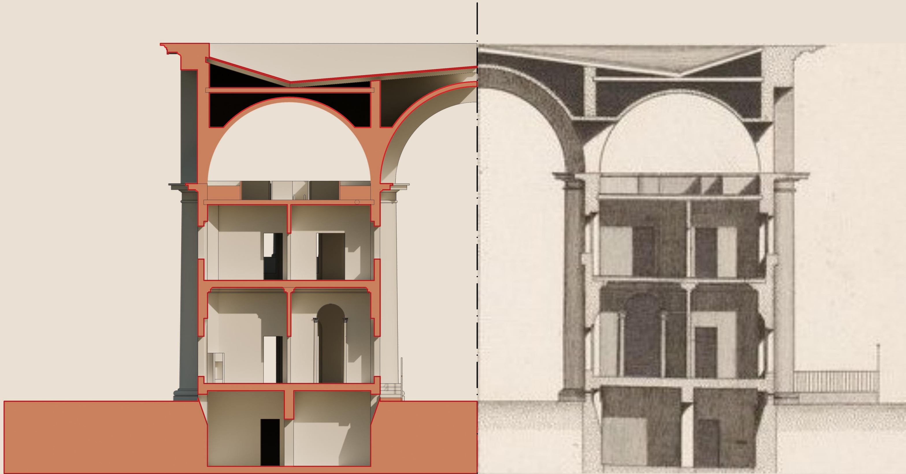
Riferimento originale di Ledoux, Sezione A-A'
