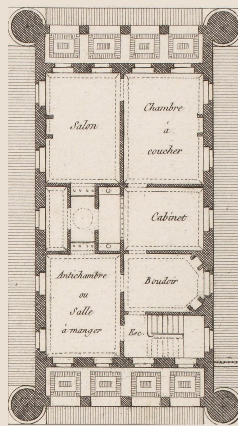
Riferimento originale di Ledoux, Pianta Piano Terra
