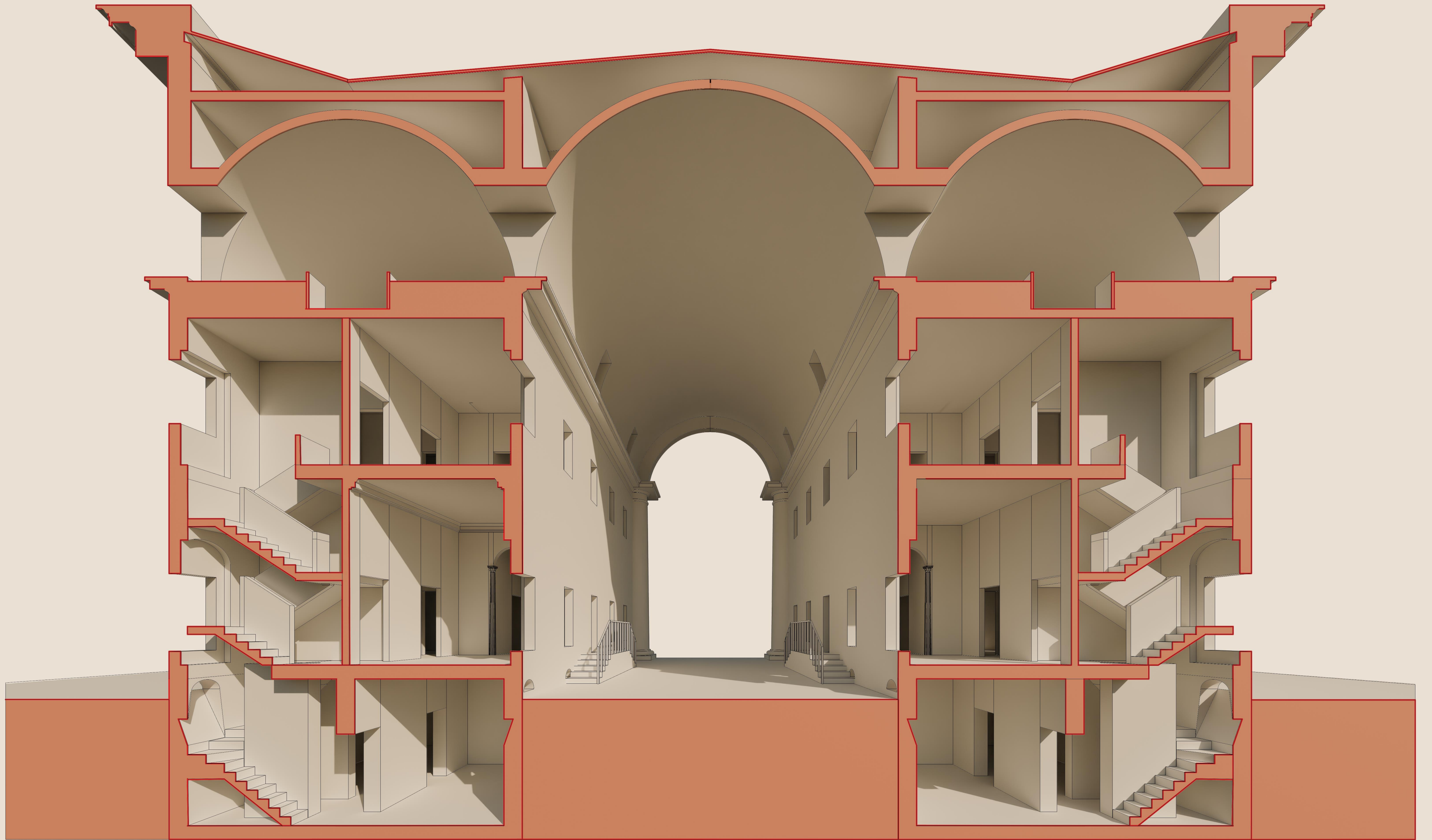
Sezione prospettica, A-A'
