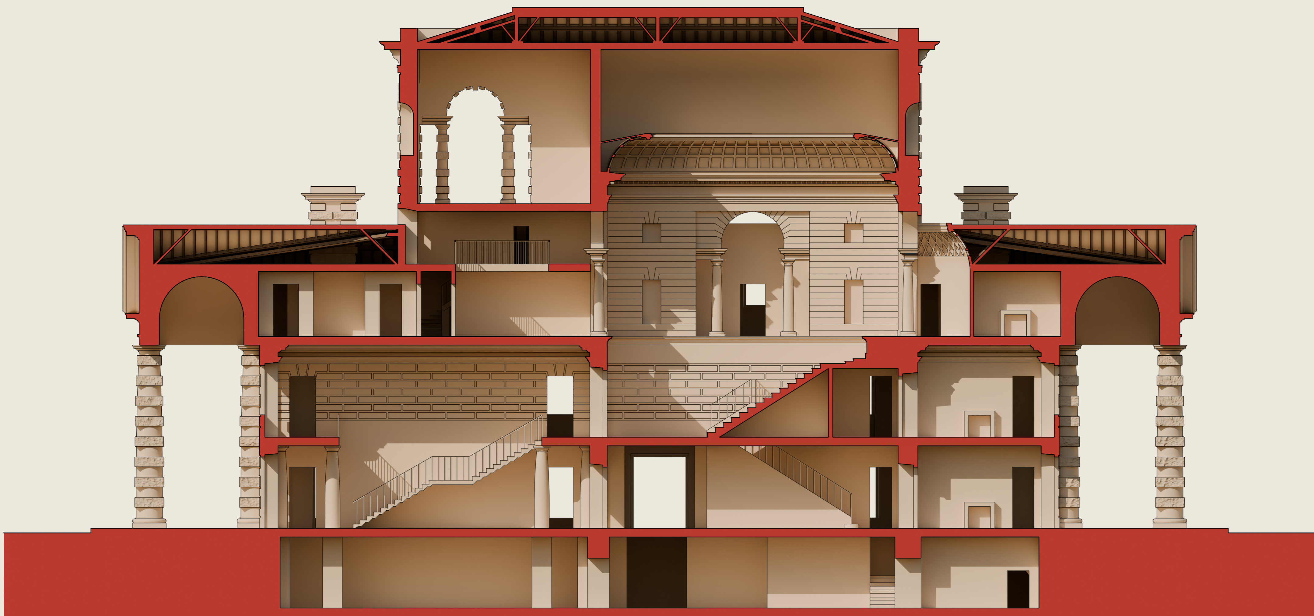
Sezione longitudinale
