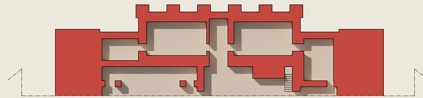
Pianta piano interrato
