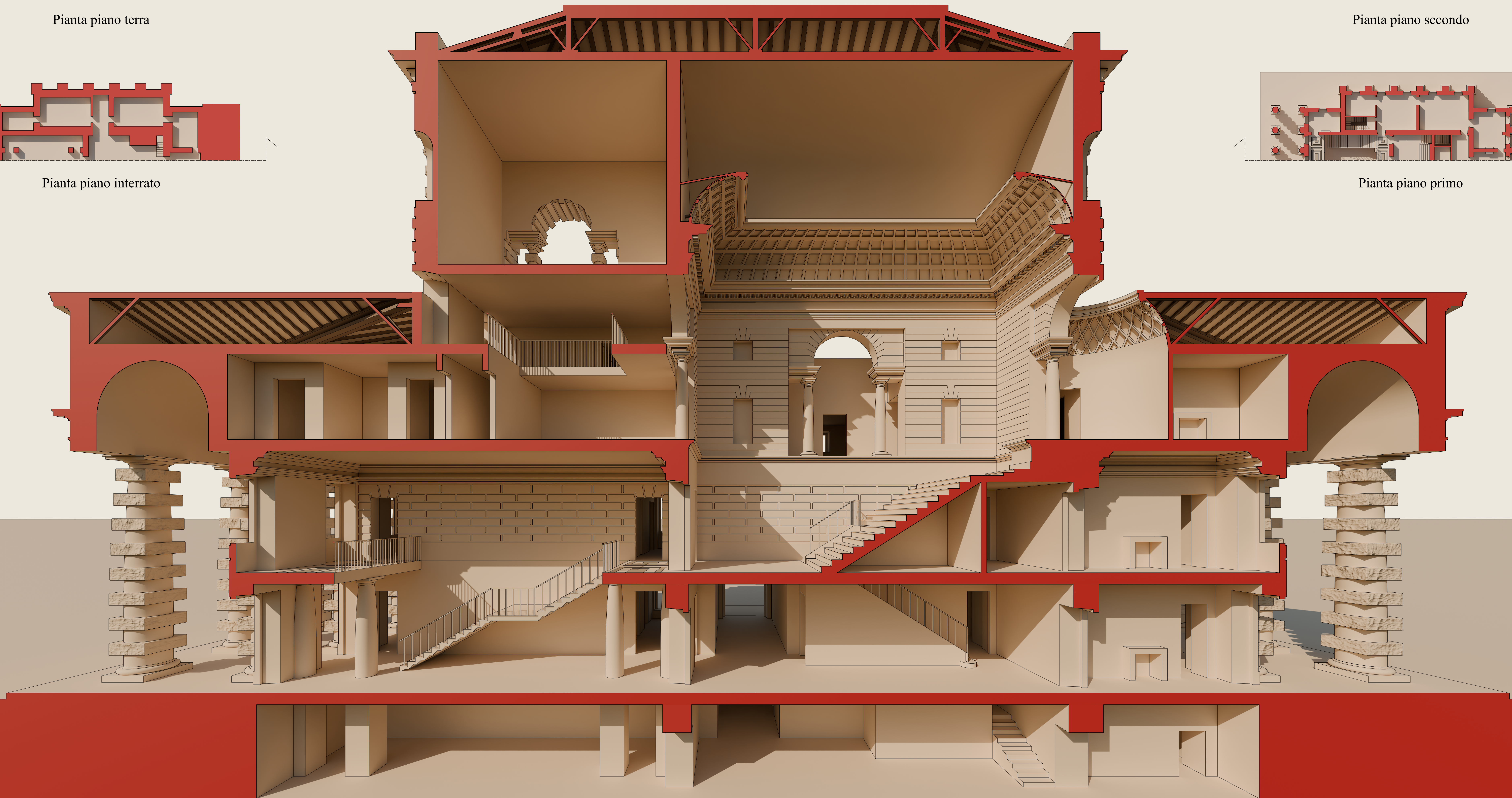
Sezione prospettica longitudinale
