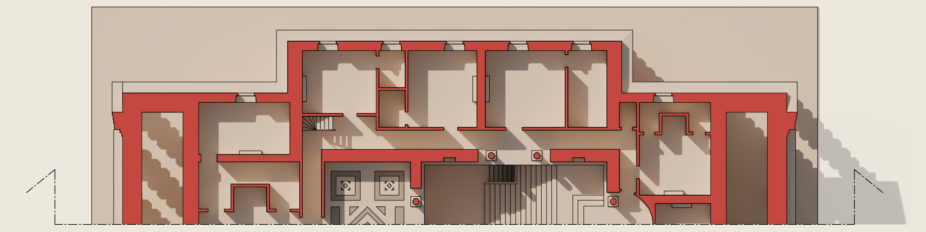
Pianta piano secondo
