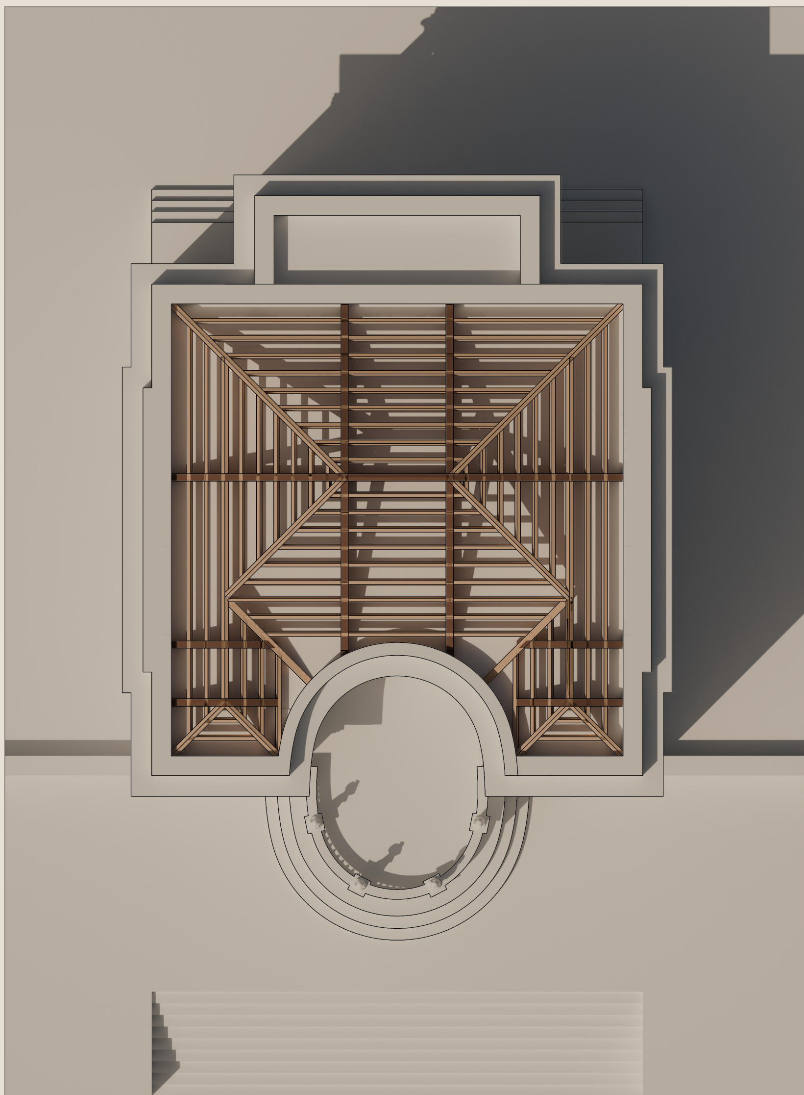
Dettaglio ortogonale della copertura
