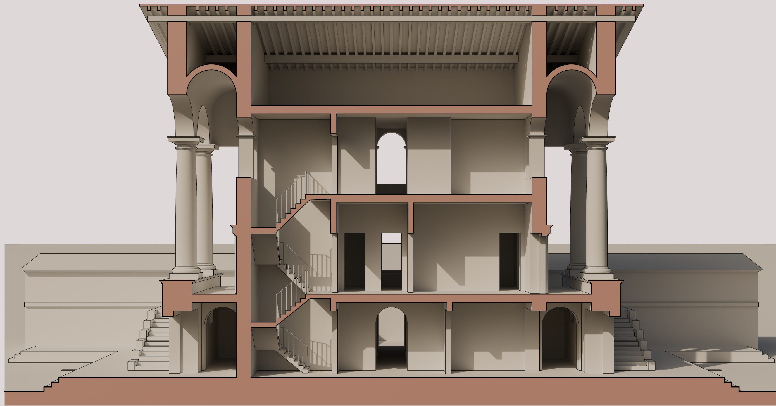
Sezione prospettica B-B'
