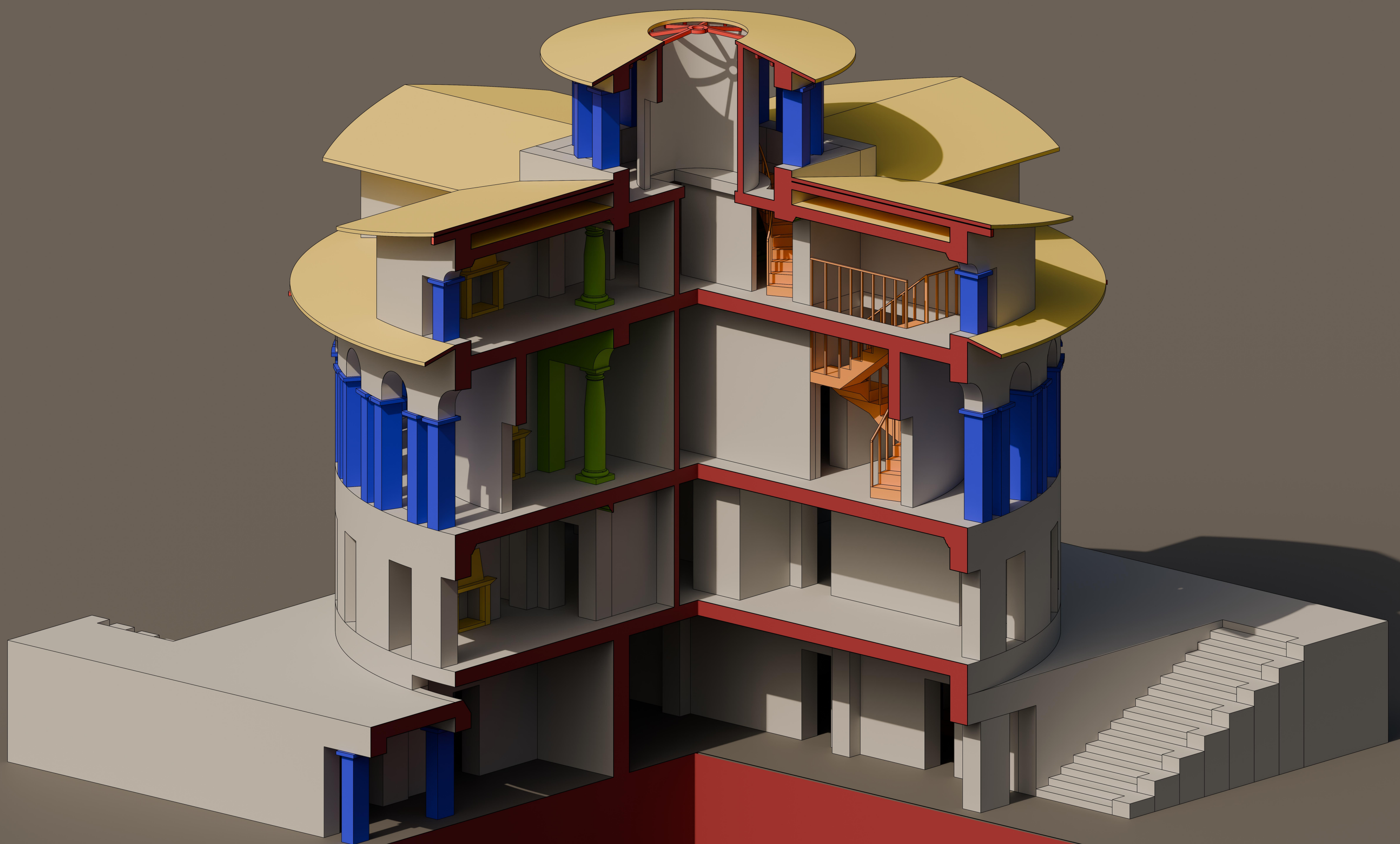
Spaccato assonometrico, scala 1:60
