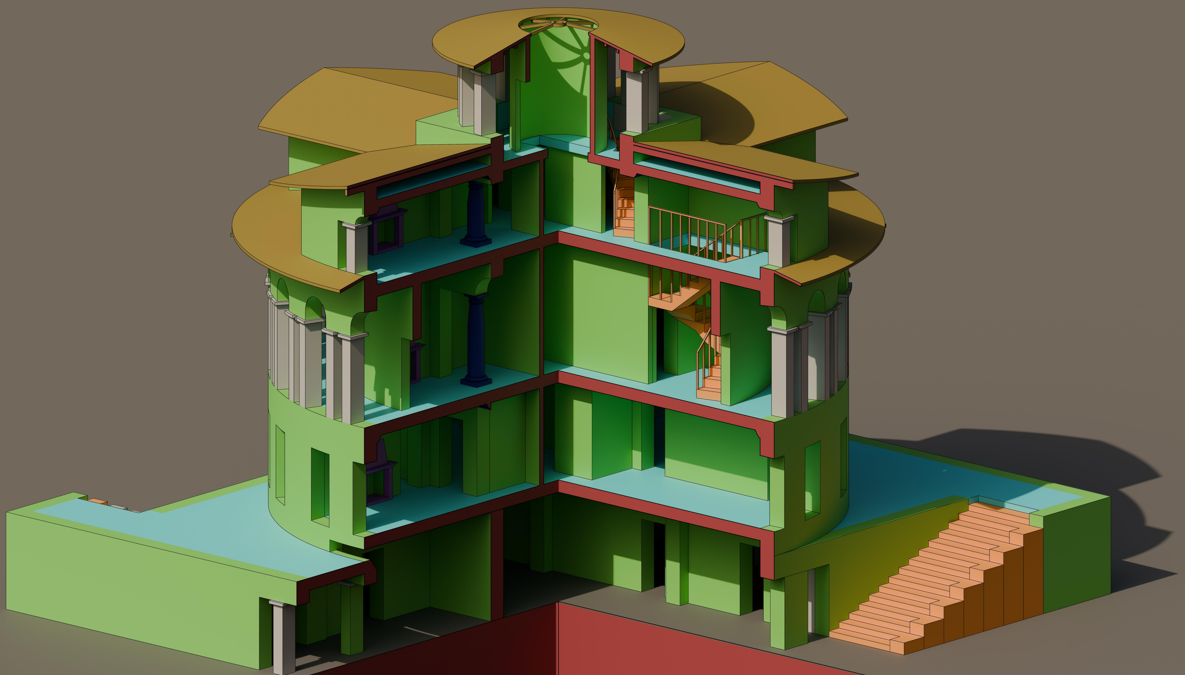
Spaccato assometrico, scala 1:60
