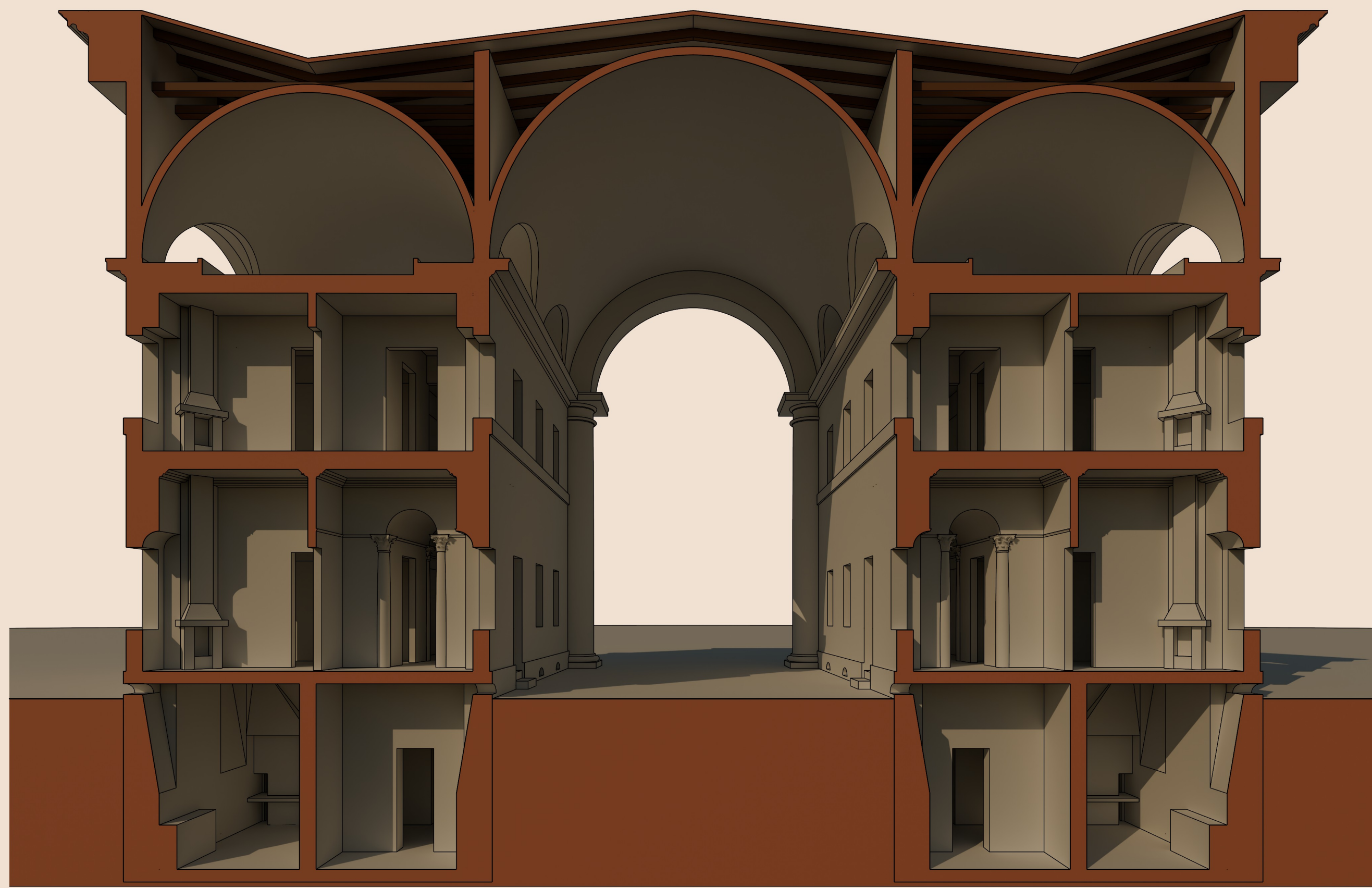
Sezione prospettica A-A'
