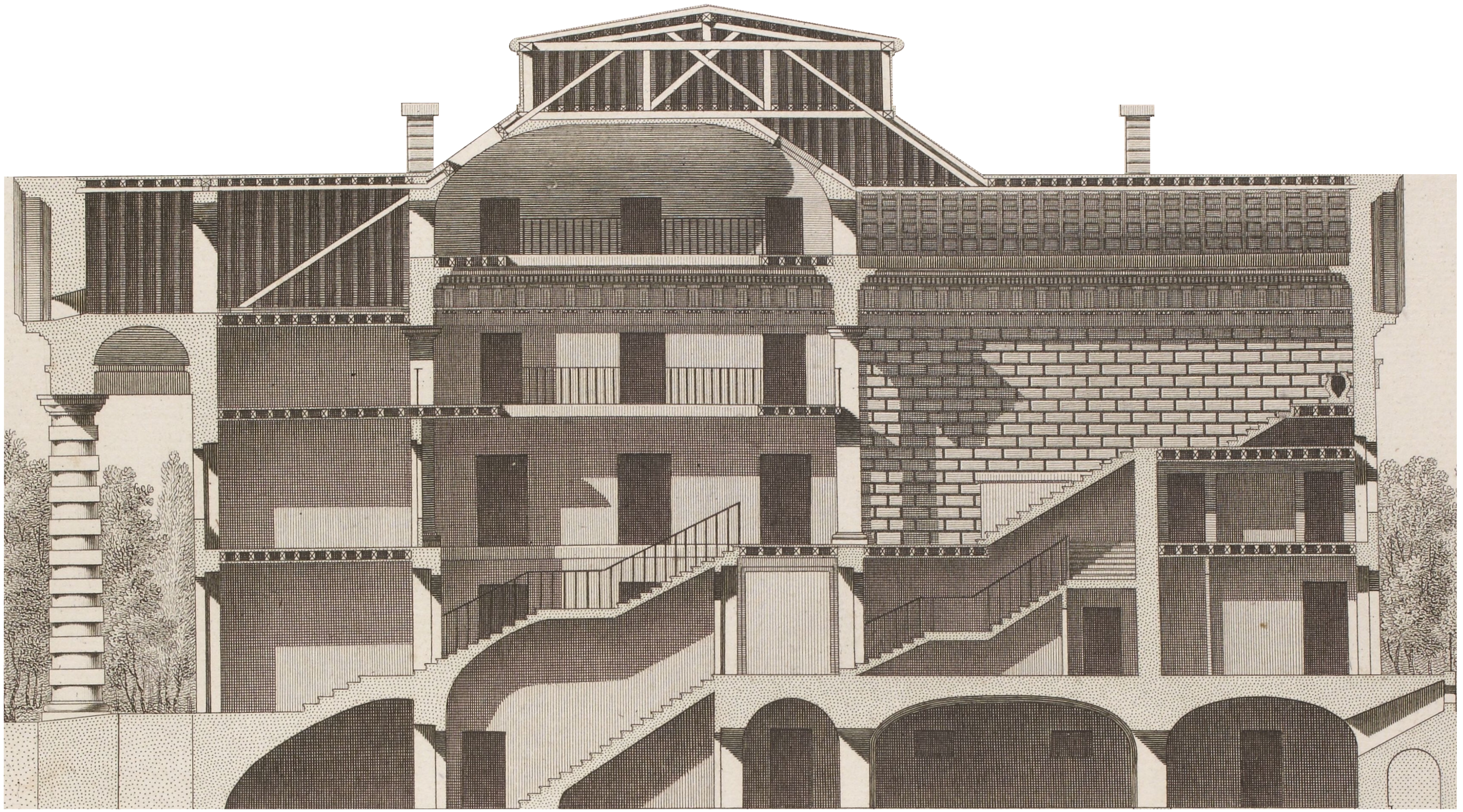
Disegno originale sezione longitudinale, scala 1:100
