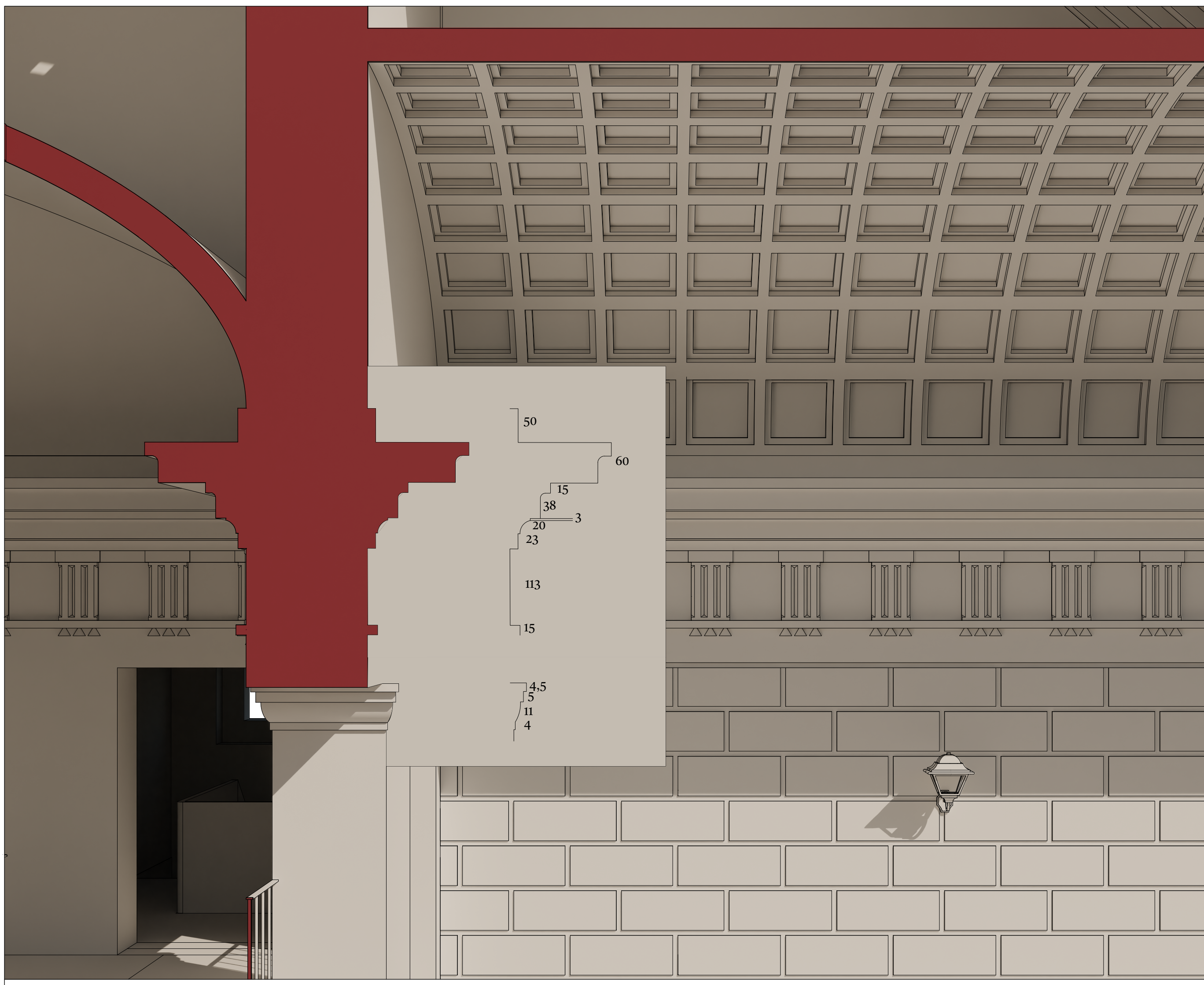
Trabeazione Interna, scala 1:20
