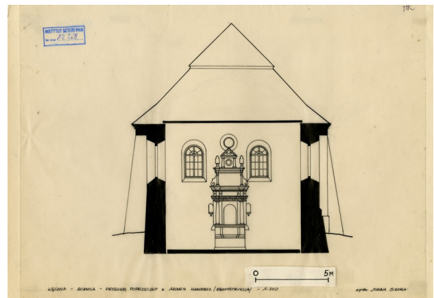
Abb. 13 Schnitt (Nord/Süd), Blickrichtung Thoraschrein, 1952
