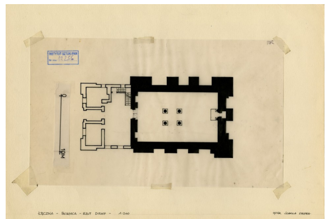
Abb. 9 Grundriss EG, 1952
