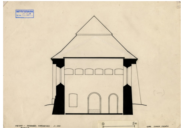
Abb. 17 Schnitt (Nord/Süd), Blickrichtung Westen, 1952
