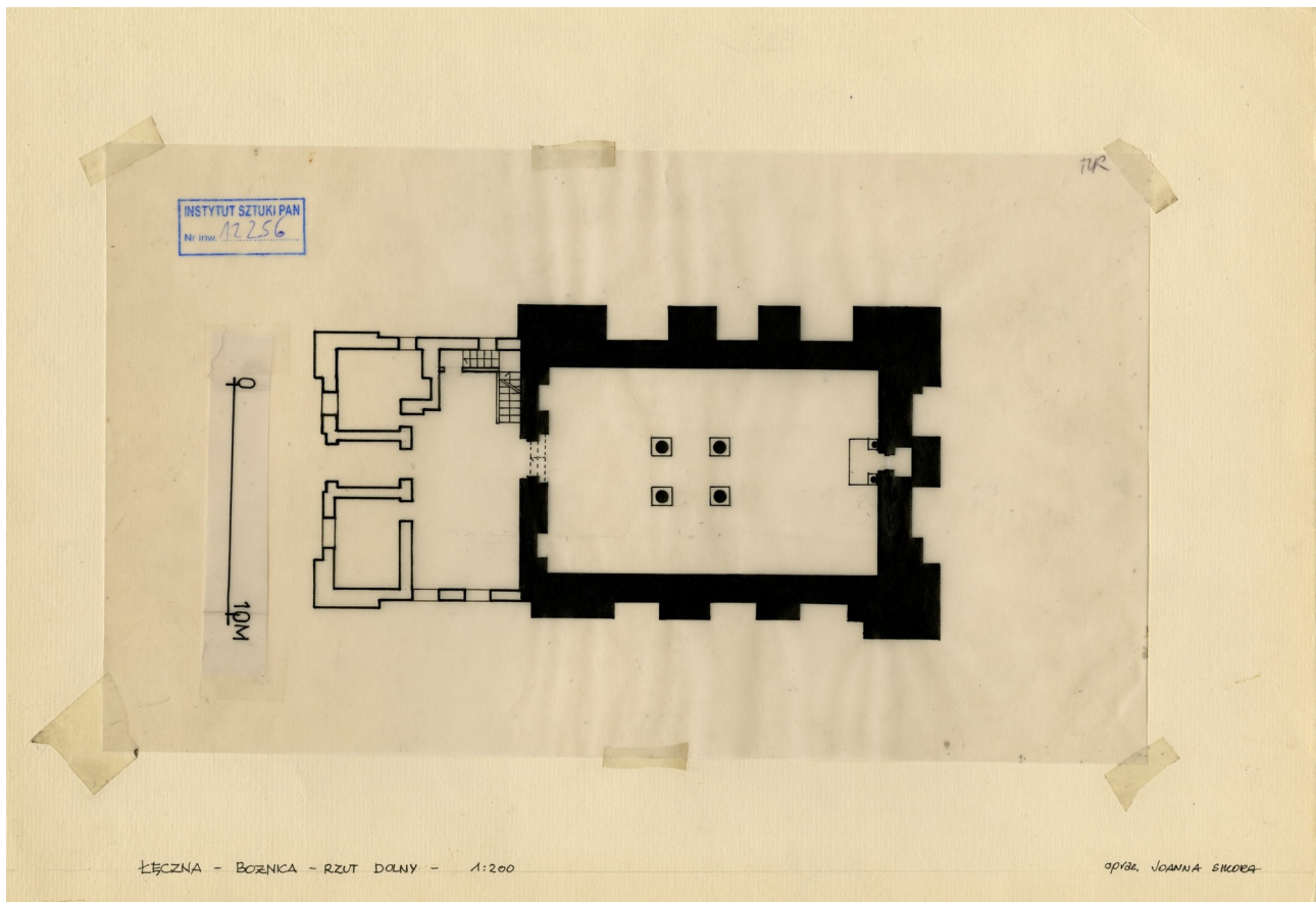
Abb. 9 Grundriss EG, 1952
