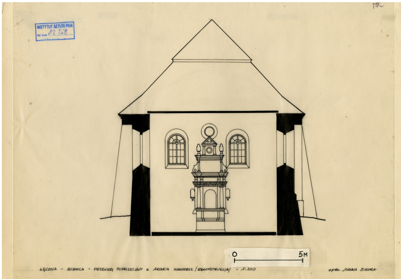
Abb. 13 Schnitt (Nord/Süd), Blickrichtung Thoraschrein, 1952
