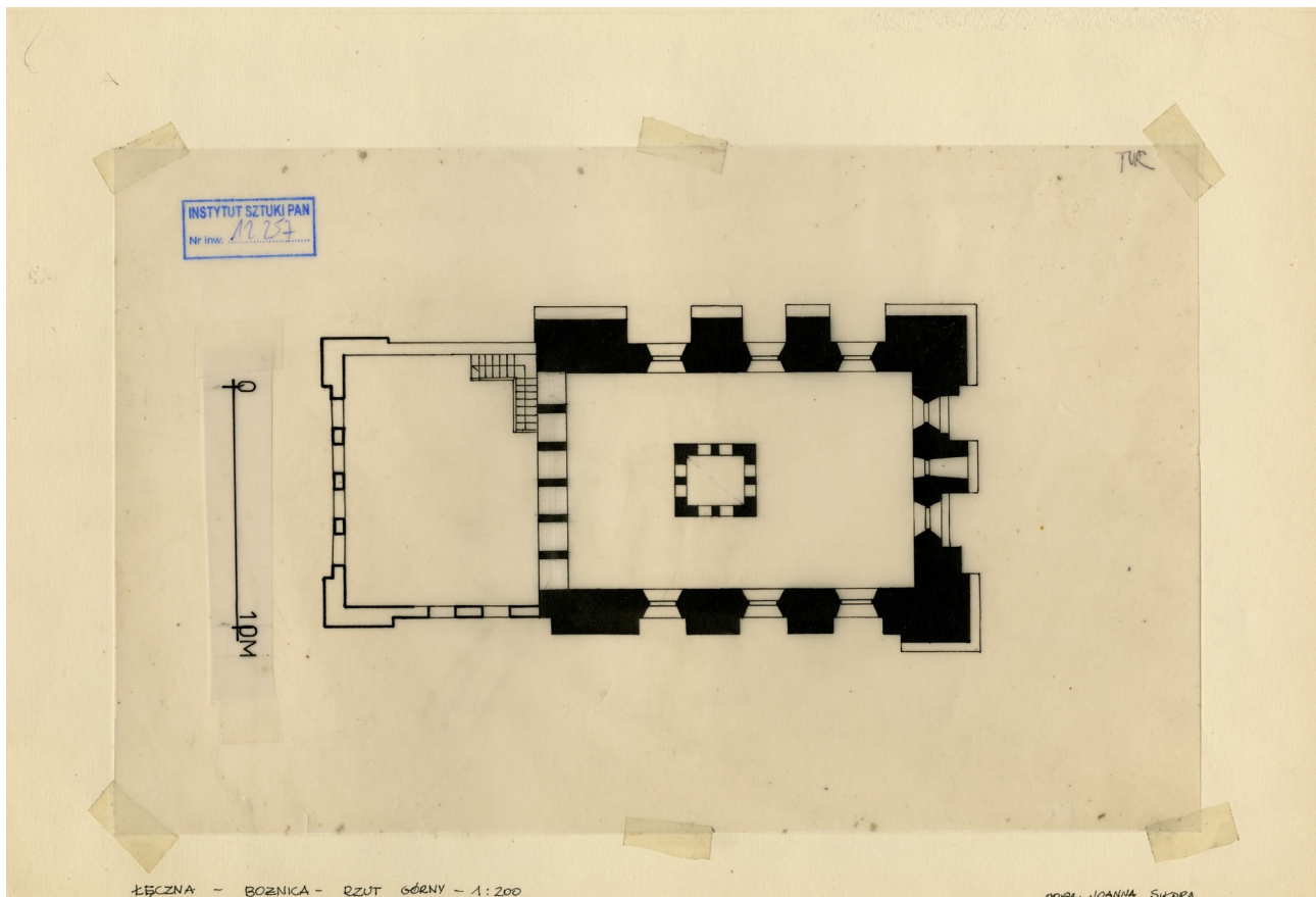
Abb. 11 Grundriss OG, 1952
