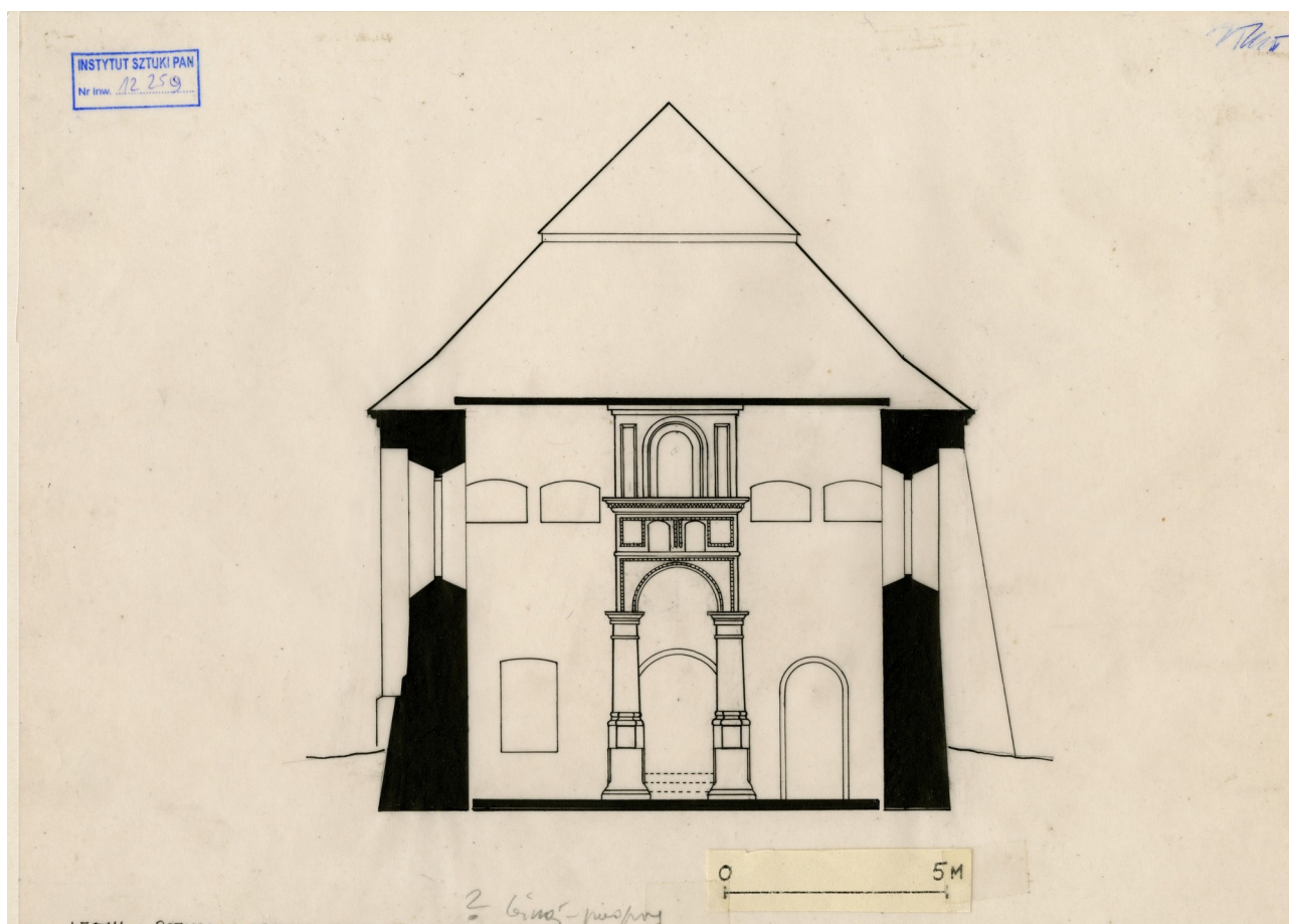
Abb. 16 Schnitt (Nord/Süd), Blickrichtung Bima, 1952
