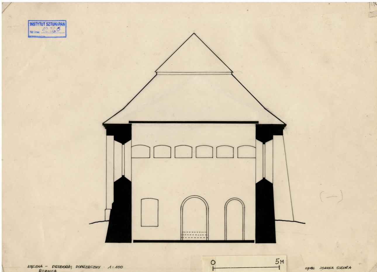
Abb. 17 Schnitt (Nord/Süd), Blickrichtung Westen, 1952
